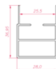
Plise - profil štoka
