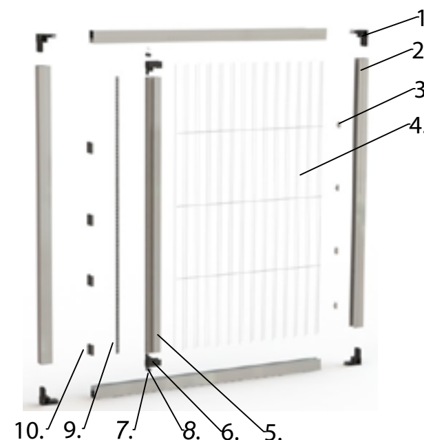
SKLOPNI PRIKAZ PLISE KOMARNIKA
