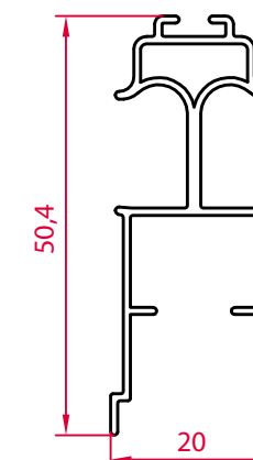
DE 1858 KRILO MALO SASH SMALL
