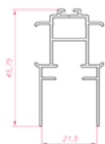
Plise - profil krila
